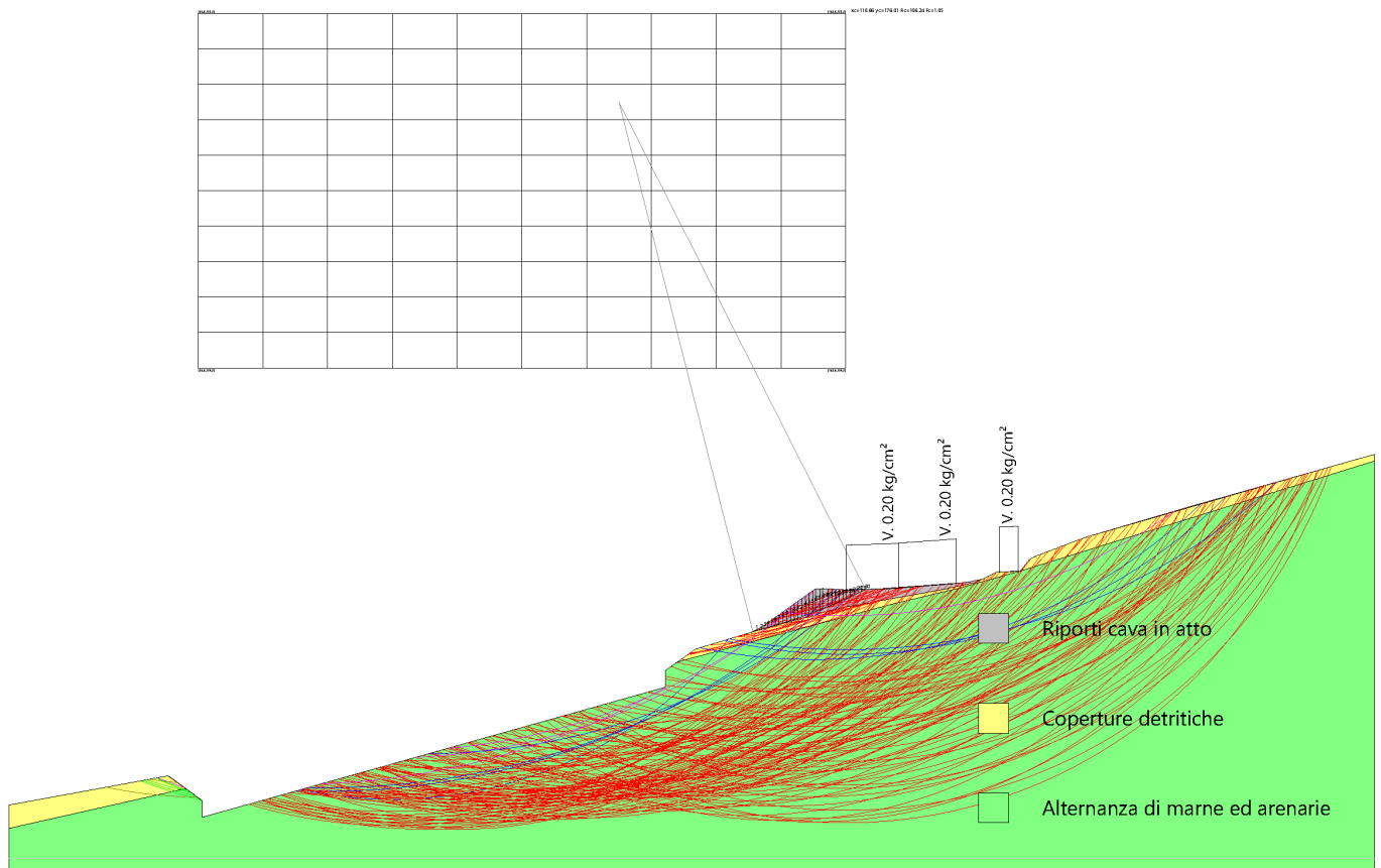
Figura rappresentante le superfici di rottura analizzate.
