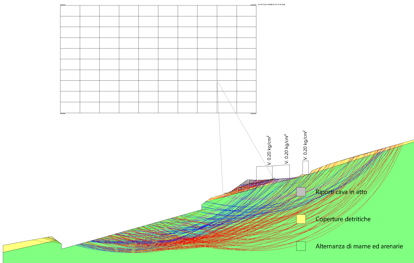
Figura rappresentante le superfici di rottura analizzate.
