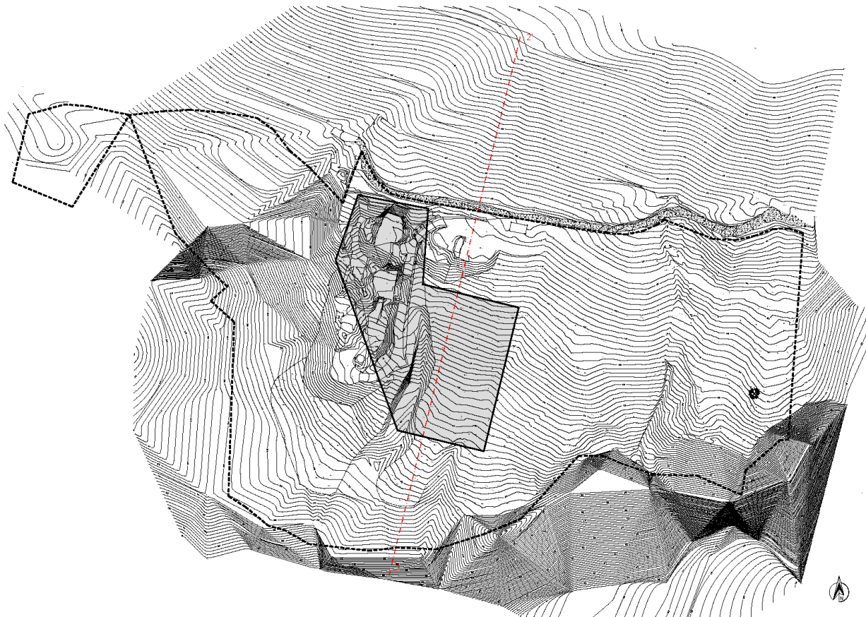
Ubicazione sezione verifica scavo 2-2'
